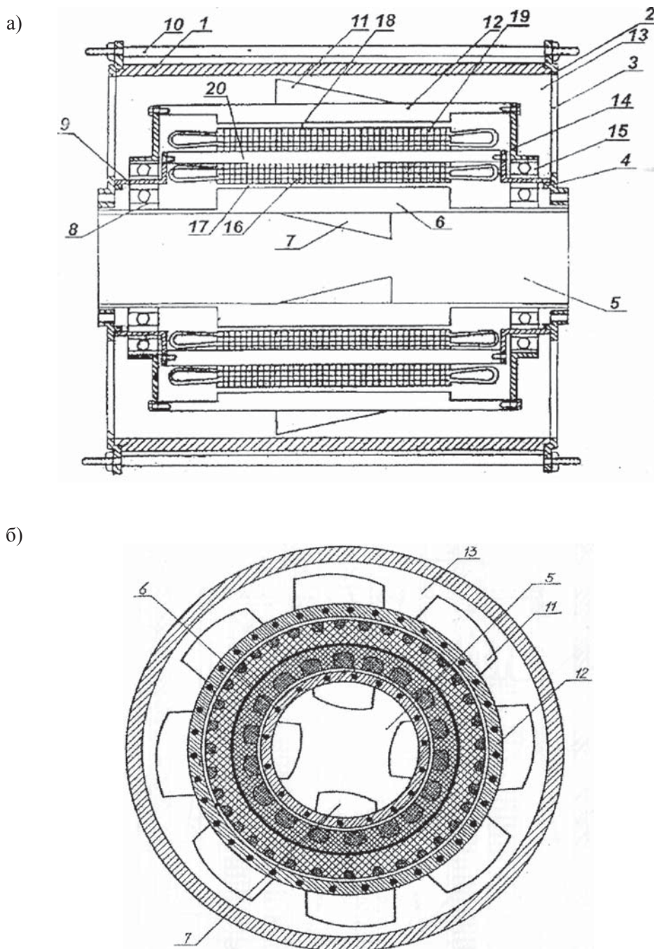
Продольный (а) и поперечный (б) разрез специального асинхронного двигателя
